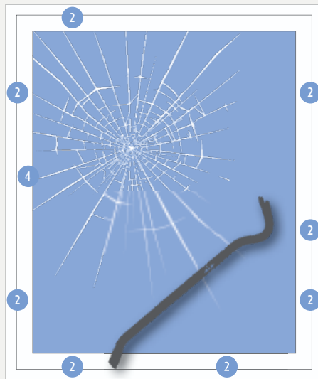
RC-3 (nur für IV88+secure) Alle Sicherheitselemente aus RC-2N. Zusätzlich durchwurfmehndes Sicherheitsglas PSA . Stahlverstärkungen im Innern gegen Aufhebeln mit schwerem Gerät.
