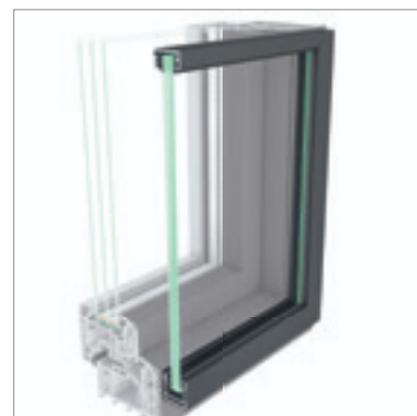
TYP 2 Vierseitiger Aluminiumrahmen. Sicherheitsverglasung 12mm stark, bis 140 cm breit.
