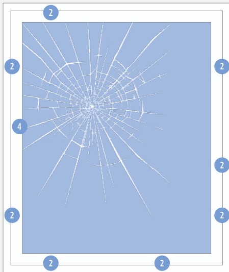
RC-2 Alle Sicherheitselemente aus RC-2N. Zusätzlich durchwurfmehndes Sicherheitsglas P4A.
