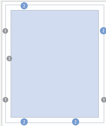
RC-1N Je nach Größe des Fensters mit 4-6 Sicherheitsschließstücken und hintergreifenden Pilzzapfen.
