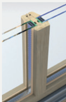
Glasteilende Sprosse Holz , 50-120 mm breit. Links die normale Sprosse, rechts Sprosse mit S-Profil.
