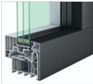
88 er Integral AUSSEN FLÄCHENBÜNDIG FENSTERFLÜGEL NICHT SICHTBAR
