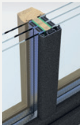
Glasteilende Sprosse Holz/Aluminium , 54, 64, 75, oder 82 mm breit.
