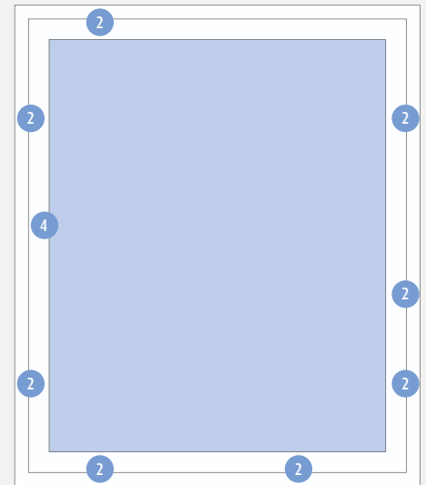
PROTECT RC-2N Je nach Fenstergröße mit 6-8 Sicherheitsschließstücken und hintergreifenden Pilzzapfen, abschließbarer Fenstergriff und Aufbohrschutz.
